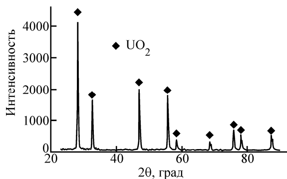
Рис. 3. Дифрактограмма UO_2 , образующегося на стенках сосуда при хранении растворов РЭ-1 и РЭ-2.
